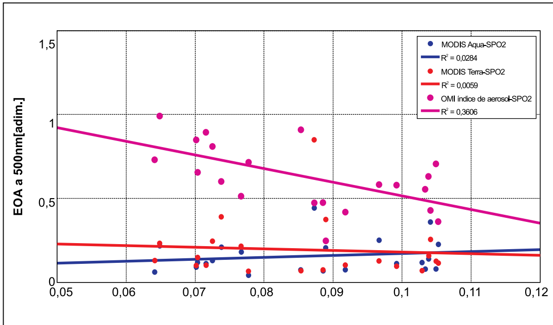
Figura N° 4: Comparación entre datos obtenidos con los sensores MODIS y OMI con el fotómetro solar SPO2-L
