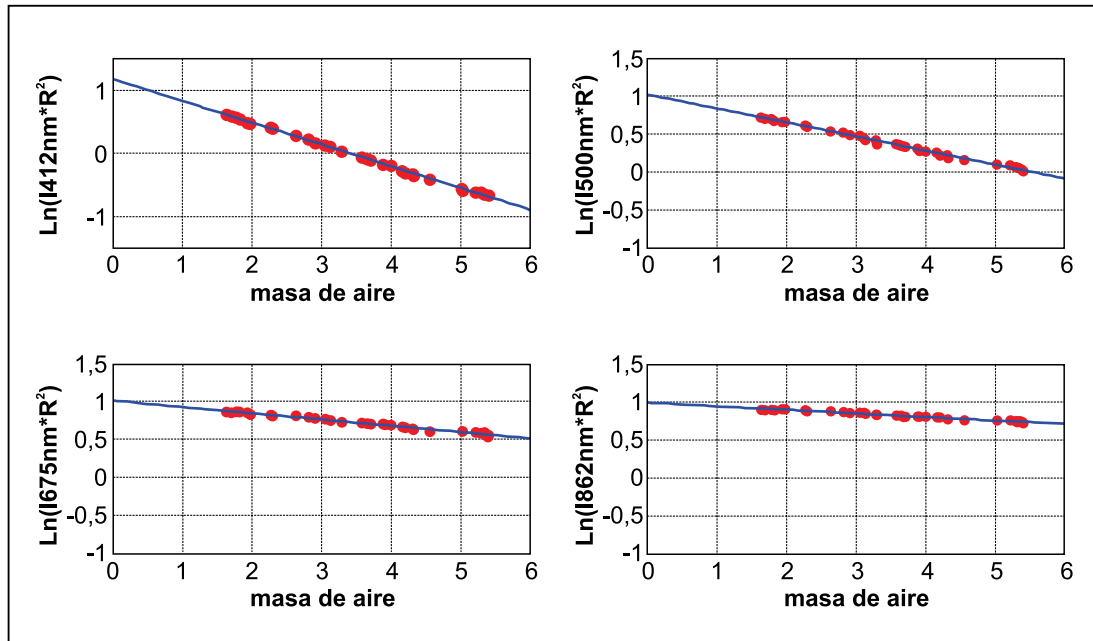
Figura N° 1: Gráfico esquemático de la curva de Langley-plot para la obtención de la intensidad en la parte superior de la atmósfera
