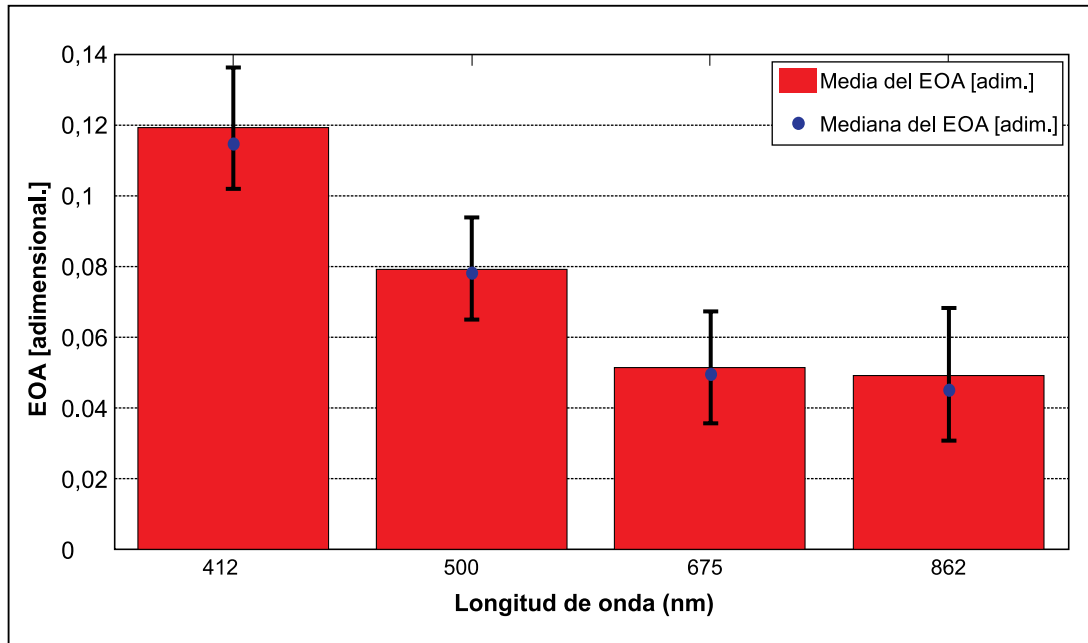
Figura N° 2: Variación del espesor óptico para cada longitud de onda
