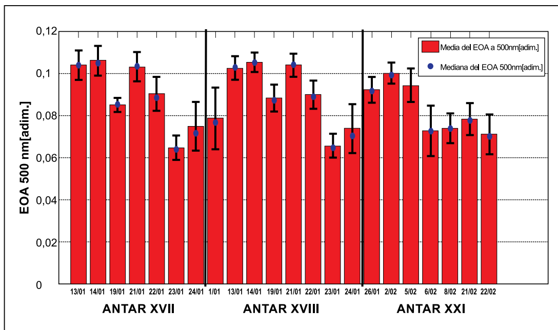
Figura N° 3: Variación diaria del EOA a 500 nm para los años de 2007, 2008 y 2013
