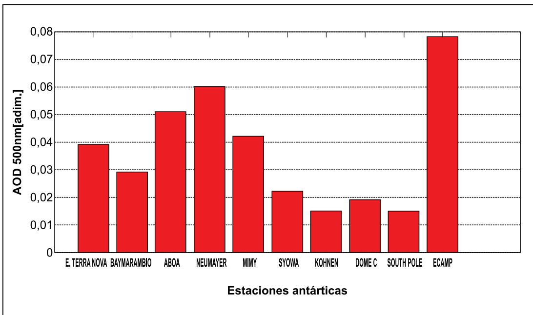
Figura N° 5: Comparación entre datos obtenidos con los sensores MODIS y OMI con el fotómetro solar SPO2-L
