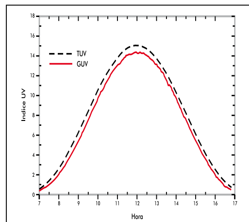
Figura Nº 2: Variación horaria del Índice UV para Huancayo. Datos radiómetro GUV y modelo TUV, 8 de setiembre del 2002.
