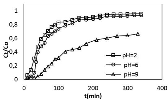
Fig. 2. Curvas de ruptura. Análisis del efecto de pH en la adsorción de AM-CA ( C_0 = 100 \text{ mg L}^{-1} , V = 20 \text{ mL min}^{-1} , Z = 10 \text{ cm} ). Fuente: Autores
