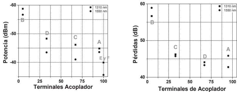
FIGURA 4. A) POTENCIA ÓPTICA EN LAS TERMINALES DE LOS ACOPLADORES A 1310 Y 1550 NM, B) PÉRDIDAS EN LAS TERMINALES DE LOS ACOPLADORES A 1310 Y 1550 NM
