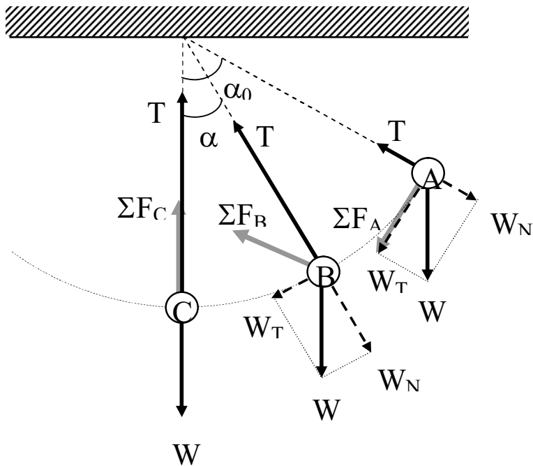
Fig. 1 - Peso de la masa oscilante, W , tensión del hilo, T , componentes normal y tangencial del peso, W_N y W_T , y fuerza total resultante, \Sigma F (y, por tanto, dirección de la aceleración correspondiente) para tres puntos representativos (A, B y C) de la trayectoria del péndulo simple.
