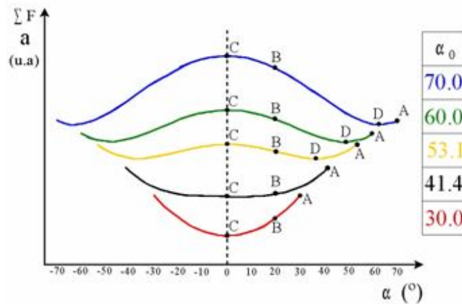
Fig. 2 - Variación con el ángulo de oscilación \alpha del módulo de la aceleración (unidades arbitrarias) y del módulo de la resultante (unidades arbitrarias) de las fuerzas que actúan sobre el péndulo, para diversas amplitudes iniciales \alpha_0 .
