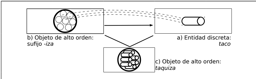
Figura 2: Esquema de composición del sufijo -iza (ejemplo: taquiza ).
