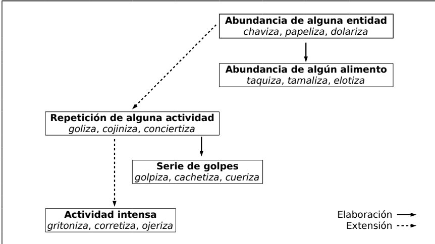
Figura 3: Red semántica del sufijo -iza.
