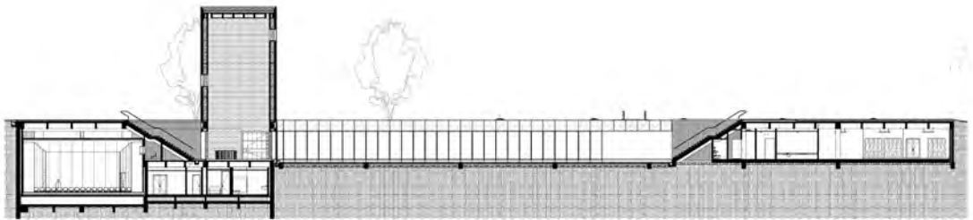
Corte B1-B1
