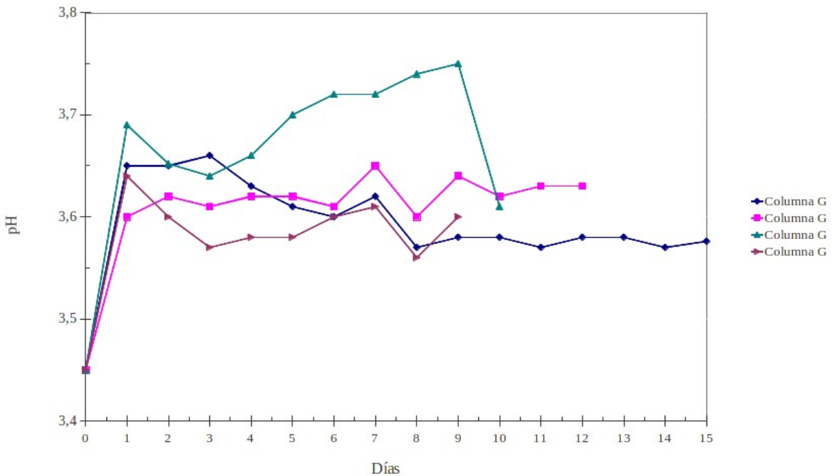
Figura 3. pH vs. Tiempo de fermentación en mostos de IT con levaduras nativas Fuente: Elaboración Propia
