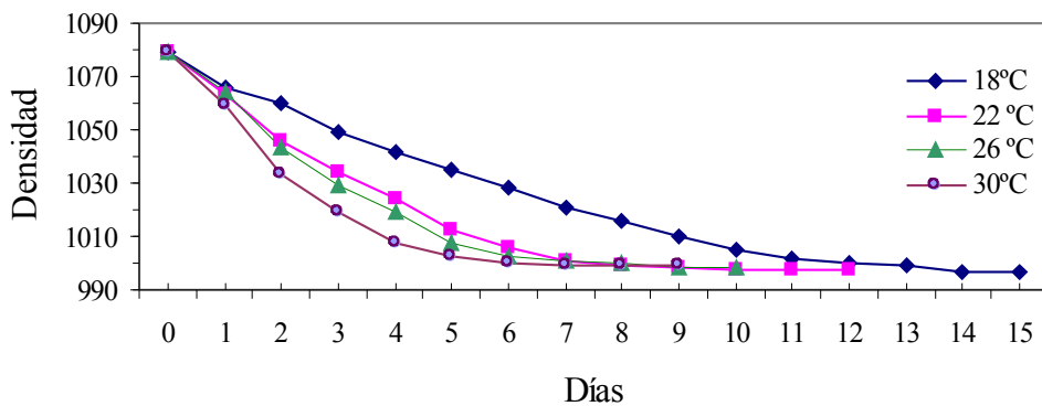
Figura 5. Densidad vs Tiempo de fermentación en mostos de IT con S. bayanus Fuente: Elaboración Propia
