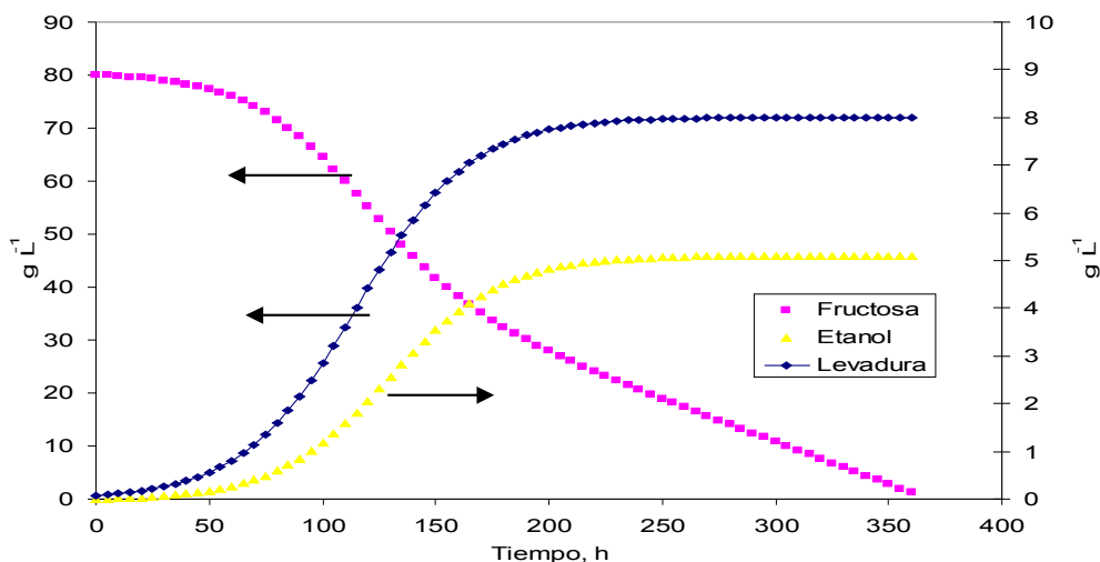
Figura 9. Curvas simuladas del consumo de fructosa por S. bayanus en el modelo logístico
