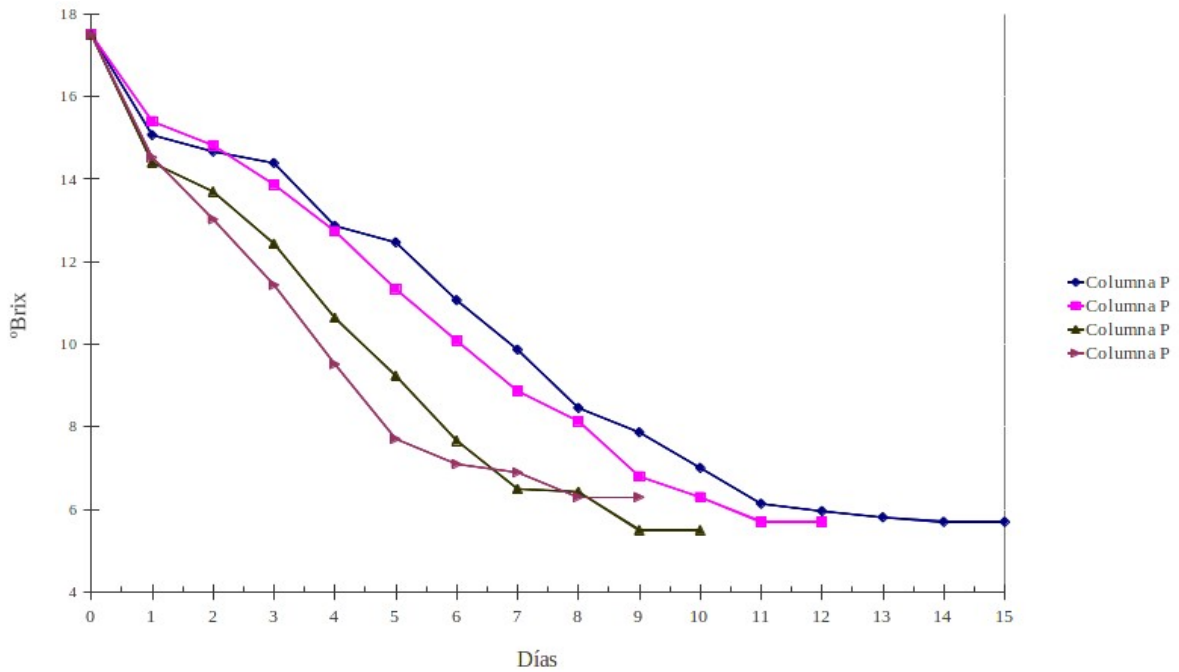
Figura 6. SST (°Brix) vs Tiempo de fermentación en mostos de IT con S. bayanus Fuente: Elaboración Propia
