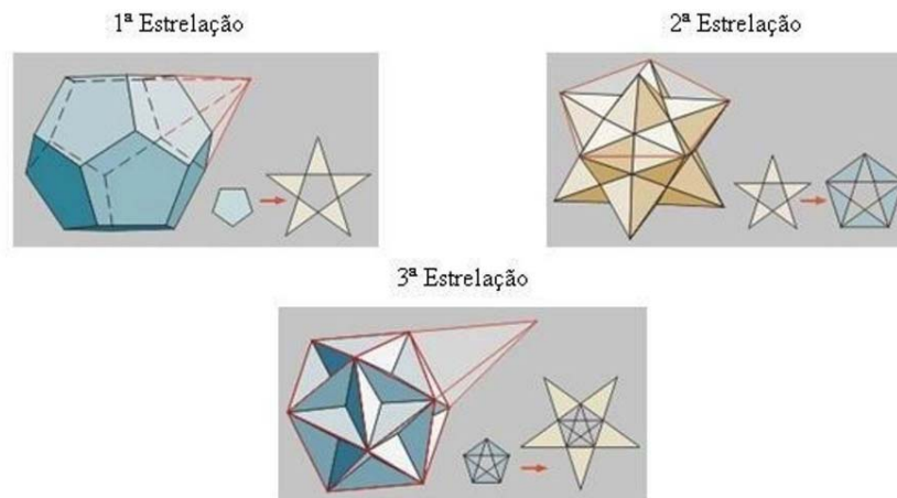
Figura 1. Formas de estrelar o dodecaedro
