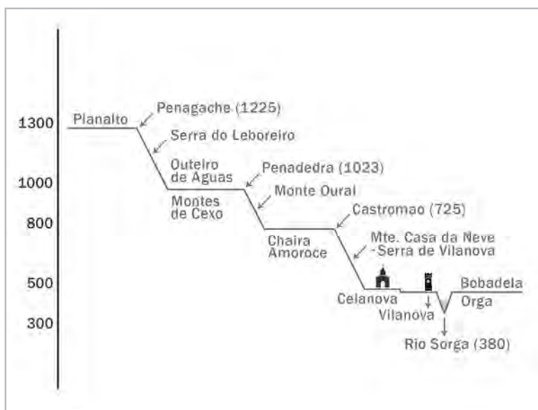
Perfil xeomorfolóxico
