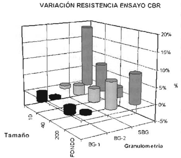
Figura No. 4. Variación de la resistencia (Ensayo C.B.R.)
