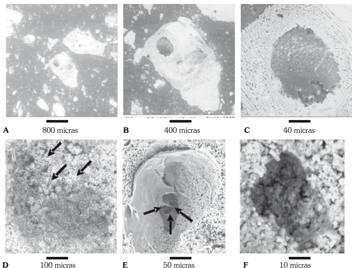
FIGURA 5. Imágenes de SEM de cultivos inducidos sobre PEBD-Cap donde se evidencia la acción de las células sobre los aglomerados grandes de CAP (A-C). Se destacan las zonas de resorción de CAP y el cambio en la morfología de los aglomerados en zonas específicas de las células, que corresponderían a zonas de sellado de los osteoclastos (Flechas D). Se destaca una laguna de resorción a 50 micras (E) y su detalle a 10 micras (F).
