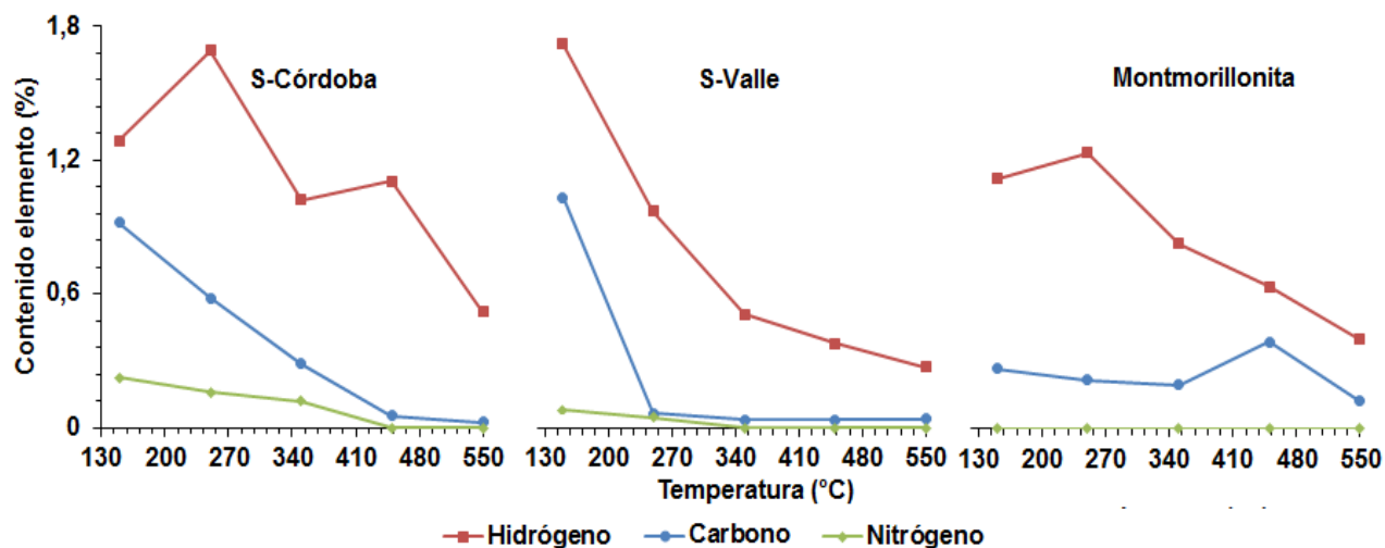
Figura 3. Contenido de elementos medidos en función de la temperatura.
