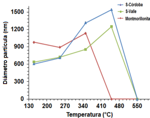
Figura 5. Diámetro de partícula en función de la temperatura.
