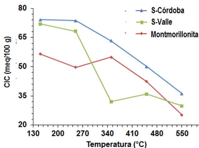
Figura 4. CIC de la fracción coloidal de los suelos en función de la temperatura.
