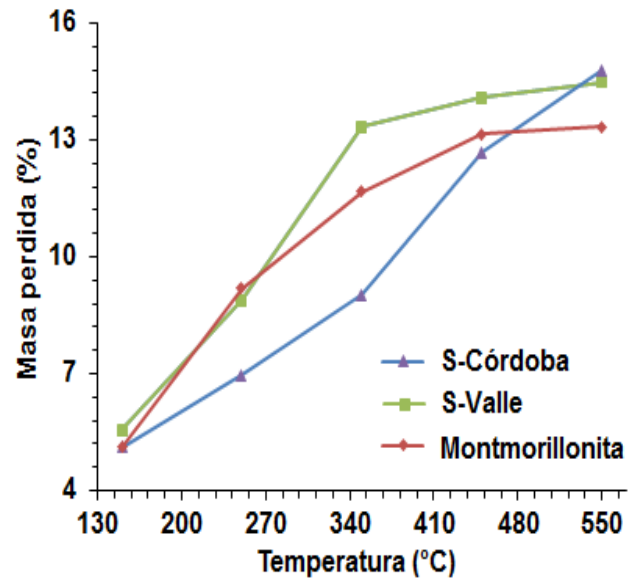
Figura 2. Masa perdida en función de la temperatura.
