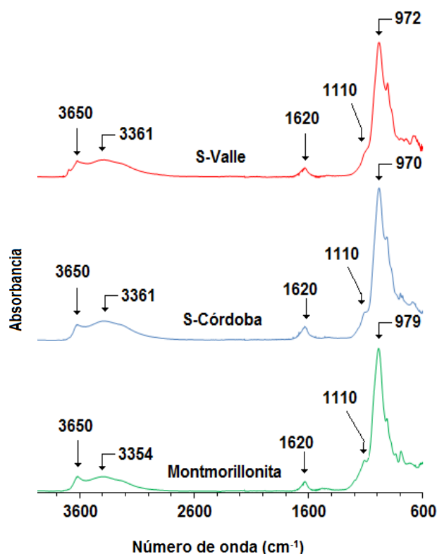
Figura 1. Espectro FT-IR/ATR de las fracciones coloidales obtenidas.
