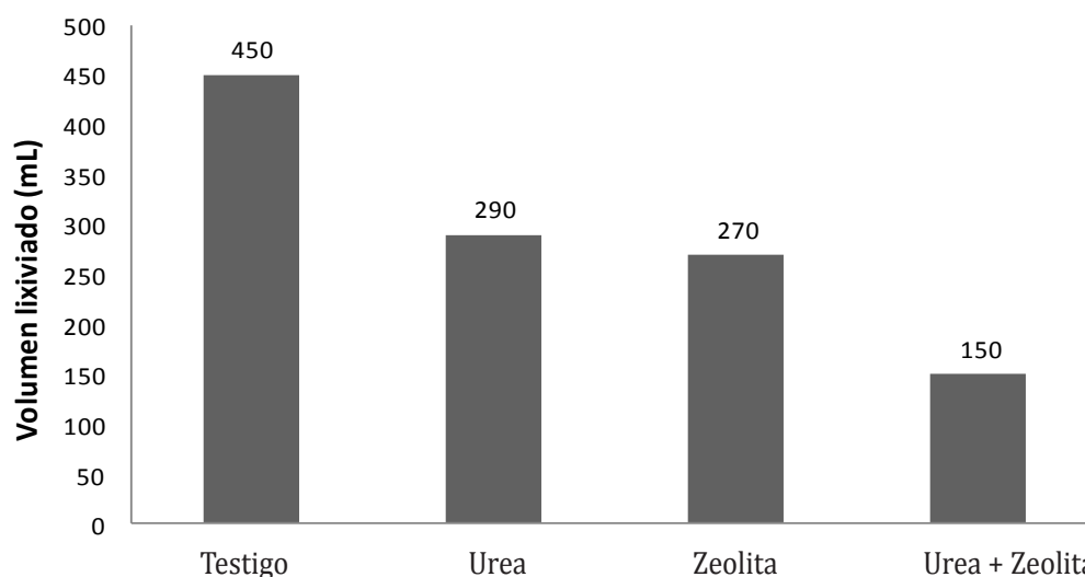
Figura 1. Efecto de la aplicación de la zeolita en combinación con urea en el volumen de lixiviados.
