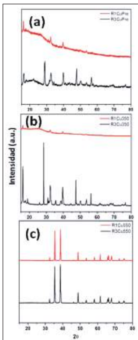
Figura 3. Comparación de la estructura cristalina del óxido de cobre (CuO) sintetizado por las rutas R1 y R3 en diferentes temperaturas. Para el CuO los planos principales son: (hkl), (2): (110) (32,3); (002), (35,5); (111),(38,7); (-202), (48,7); (202), (58,2);(-113),(62,4) y (-311), (68,4). Fuente: autores
