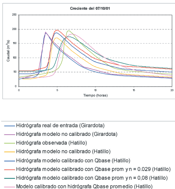
Figura 3. Comparación de las hidrógrafas de caudal para la creciente del 07/10/01 en fronteras del tramo
