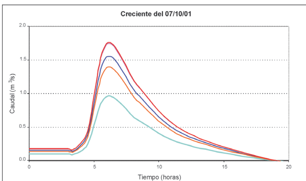
Figura 5. Hidrógrafas de aporte de caudal lateral para los 5 subtramos de Girardota-El Hatillo
