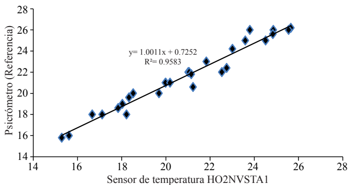
Figura 6. Relación entre en la temperatura de sensor (HO2NVST1) y el termómetro seco del psicrómetro. Figure 6. Relationship between the temperature sensor (HO2NVST1) and dry thermometer of the psychrometer.
