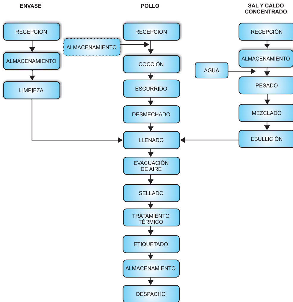
Figura 1. Diagrama de flujo de la línea de pechuga desmechada enlatada
