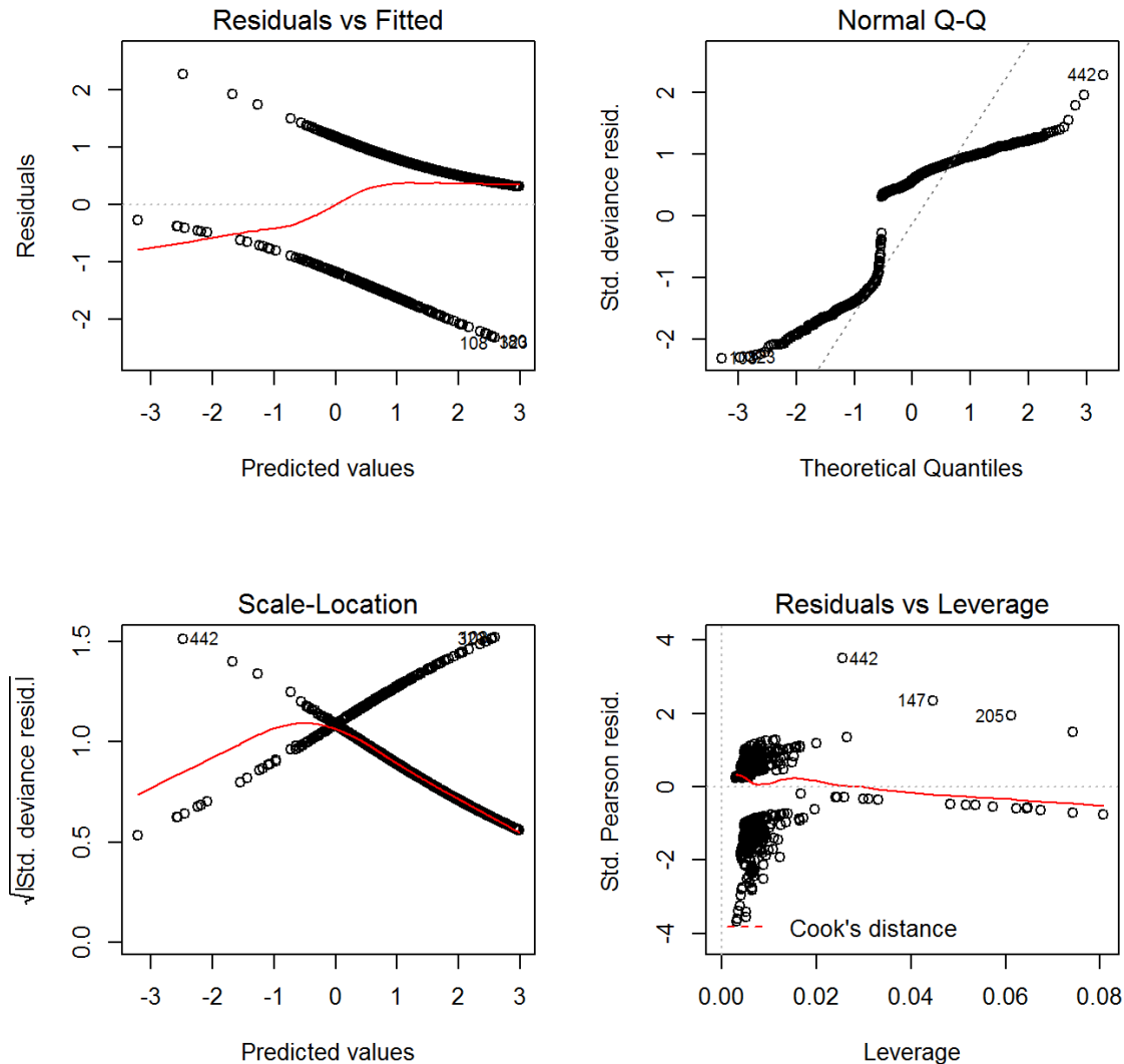
Figura 3. Serie de gráficos obtenidos en el análisis de residuos.
