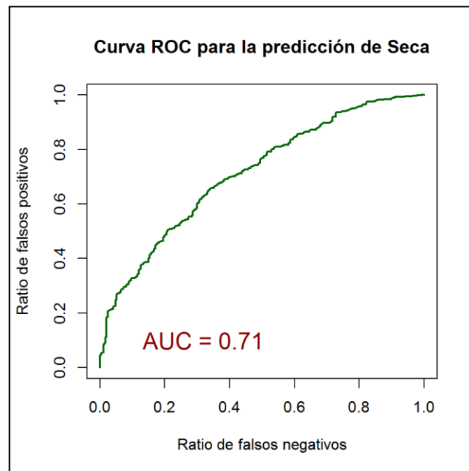
Figura 4. Curva ROC para la predicción de Seca.
