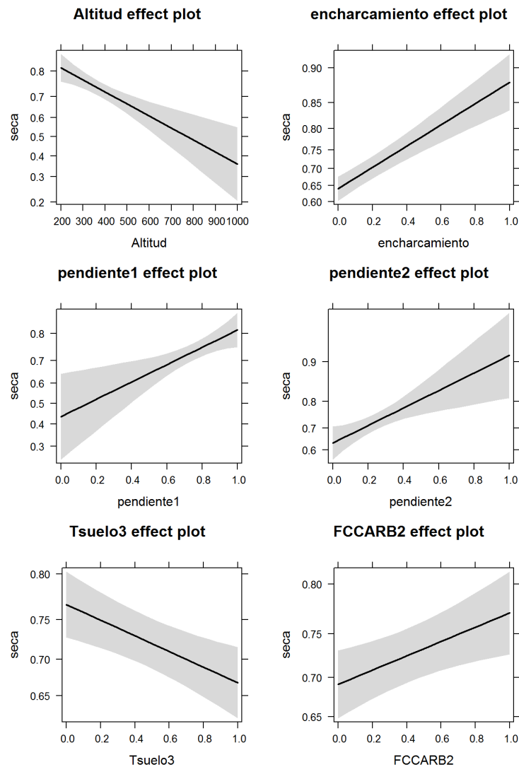
Figura 2. Serie de gráficos de influencia de las variables en el fenómeno Seca según el modelo propuesto.
