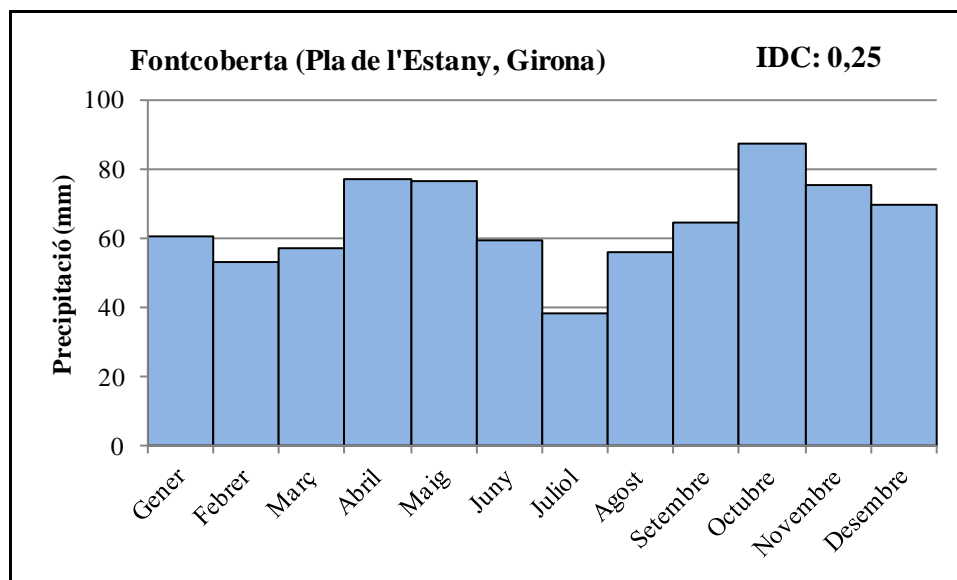
Figura 5. Histograma de la pluviometria anual a Fontcoberta, (1981-2010)
