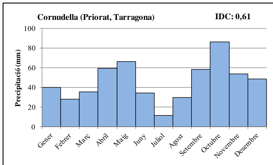
Figura 4. Histograma de la pluviometria anual a Cornudella, (1981-2010)
