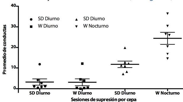
Figura 4 Operantes durante la supresión de reforzadores para cada cepa en las sesiones diurnas y nocturnas
