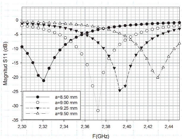
Figura 4. Efecto en la magnitud del coeficiente de reflexión S_{11} para diferentes valores del radio interior a , con b=26.3 mm y p=13.4 mm. Fuente: Los Autores.
