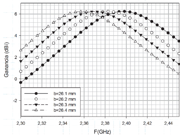
Figura 6. Efecto en la magnitud de la ganancia para diferentes valores del radio exterior b , con a=9 mm y p=13.4 mm. Fuente: Los Autores.
