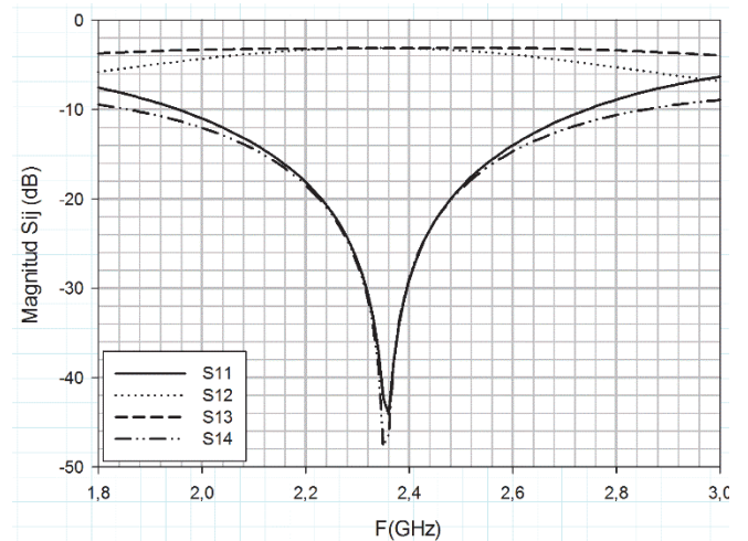
Figura 9. Resultados de las simulaciones de los parámetros de dispersión S_{11} , S_{12} , S_{13} y S_{14} para el híbrido de 90°. Fuente: Los Autores.
