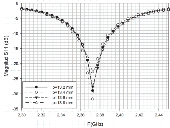
Figura 5. Efecto en la magnitud del coeficiente de reflexión S_{11} para diferentes valores del radio de excitación p , con a=9 mm y b=26.3 mm. Fuente: Los Autores.
