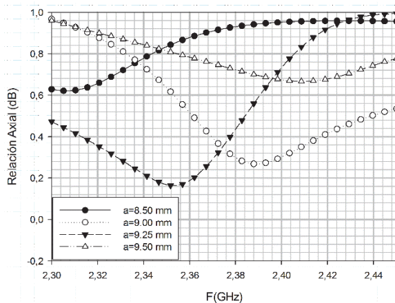
Figura 7. Efecto en la magnitud de la relación axial para diferentes valores del radio interior a , con b=26.3\text{ mm} y p=13.4\text{ mm} . Fuente: Los Autores.
