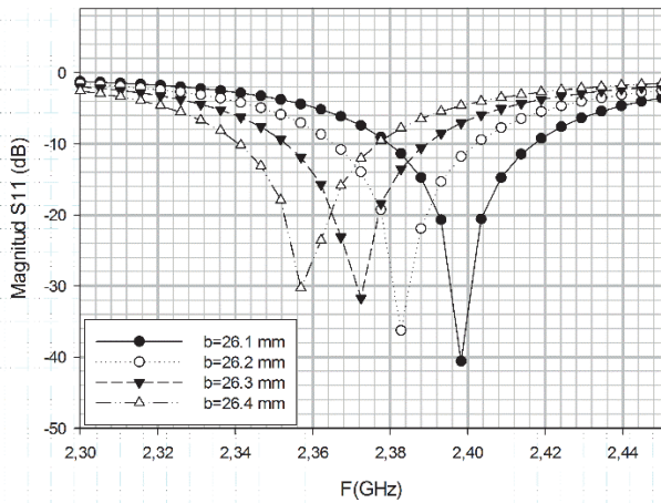
Figura 3. Efecto en la magnitud del coeficiente de reflexión S_{11} para diferentes valores del radio exterior b , con a=9 mm y p=13.4 mm. Fuente: Los Autores.
