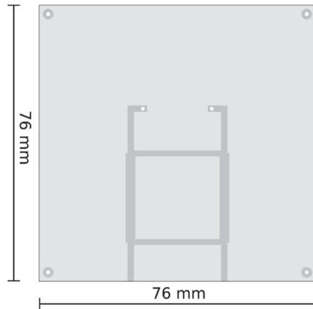
Figura 8. Vista superior del híbrido de 90° con un plano de masa de 76\text{ mm} \times 76\text{ mm} . Fuente: Los Autores.
