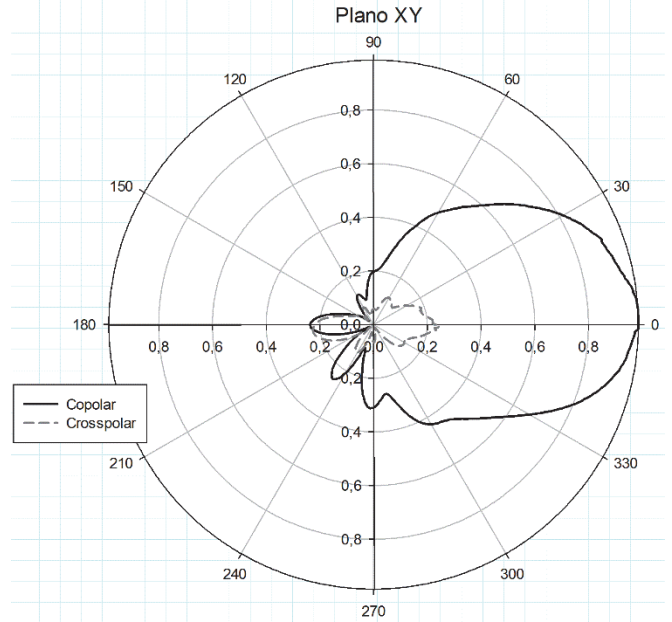
Figura 16. Resultados de las medidas de los diagramas de radiación Copolar y Crosspolar en el plano XY. Fuente: Los Autores.
