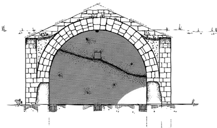
Sección transversal
