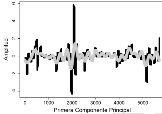
Figura 4. Primera componente principal para El-Salitre, serie original línea negra, representación con 20 armónicos relevantes, línea gris.
