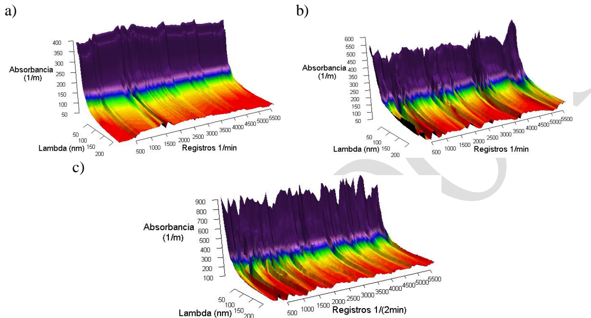
Figura 1. Series temporales de absorbancia UV-Vis para El-Salitre (a), EBG (b) y San-Fernando (c). (adaptado de [40]).
