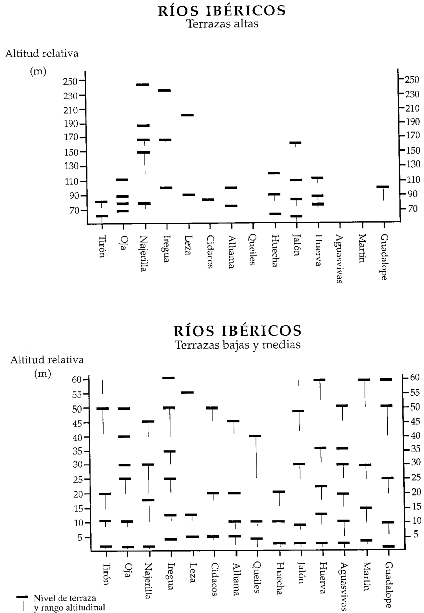
Figura 3.- Secuencias de niveles de terrazas de los principales ríos ibéricos en la Depresión del Ebro. Fuente de los datos de altitud relativa: Tirón, Oja, Najerilla e Iregua, JULIÁN (1997); Leza y Cidacos, GONZALO (1981); Alhama y Queiles, LERÁNOZ (1993); Huecha, PELLICER (1984); Jalón y Huerva, SORIANO (1986); Aguasvivas, ECHEVERRÍA (1984); Martín y Guadalupe, JULIÁN (1996).
