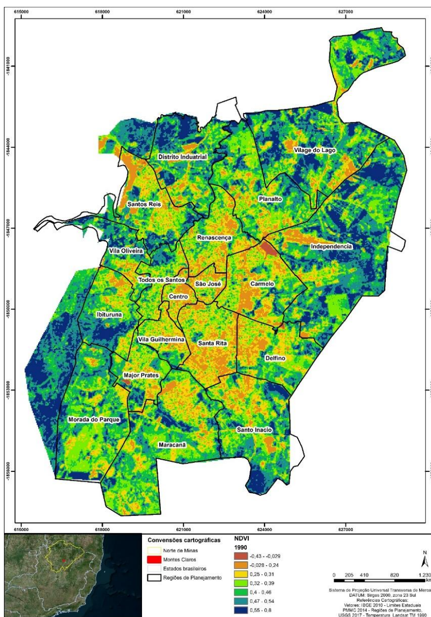
Figura 02 - NDVI 1990.
