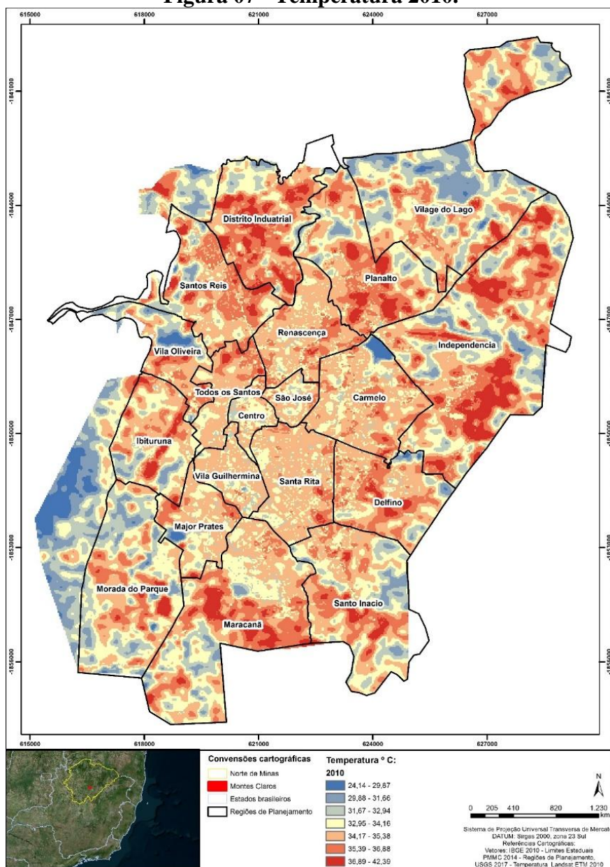
Figura 07 - Temperatura 2010.
