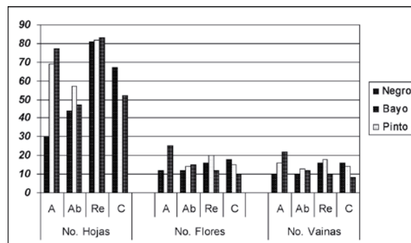
Figura 2. Número de hojas, flores y vainas de cada variedad de frijol con los diferentes tratamientos a los 68 días. A; aislado A, Ab; aislado Ab, Re; cepa de Rhizobium etli , C; control sin inóculo. Cada barra representa la cantidad promedio de 20 plantas analizadas en los diferentes tratamientos.
