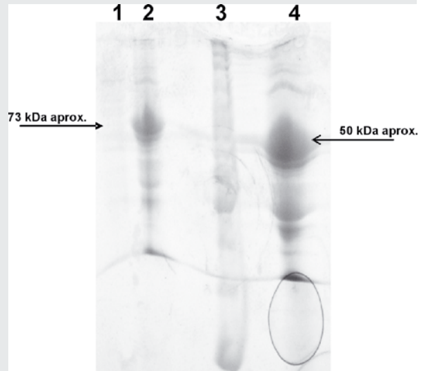
Figura 5. Proteínas totales de vainas de frijol Bayo tratadas con diferentes aislados. 1) Control sin inocular, 2) Con la cepa Re; existe una expresión de una proteína de aprox. 73 kDa. 3) MPM y 4) Con el aislado A, donde se presenta una sobreexpresión de una proteína de aproximadamente 50 kDa.
