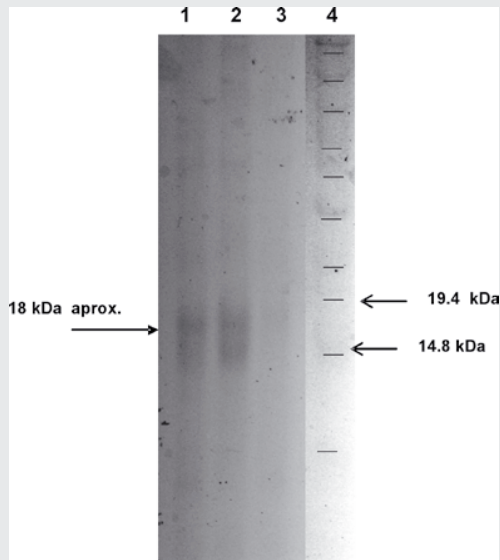
Figura 4. Electroforesis de proteínas totales de hojas de frijol Bayo tratado con diferentes aislados. 1) Muestra de proteínas de hojas de plantas tratadas con el aislado A, 2) Proteínas con el aislado Ab., 3) Control, sin inocular y 4) Marcador de peso molecular (MPM). Se observa en los carriles 1 y 2 una expresión de una proteína de aproximadamente 18 kDa.
