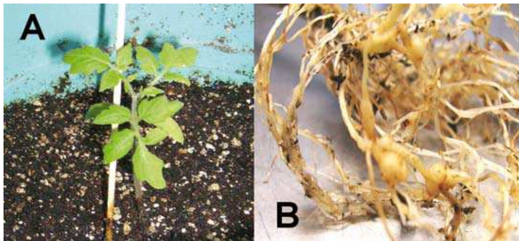
Figura 6. Efecto del aislado A en el crecimiento y nodulación de plantas jitomate Bola A) Crecimiento de la planta a los 68 días y B) Nódulos en raíces.
