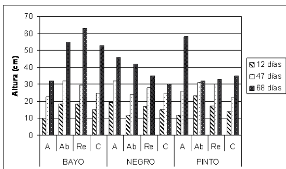
Figura 1. Altura de plantas de frijol tratadas con inóculos de rizobacterias en diferentes tiempos. A; aislado A, Ab; aislado Ab, Re; cepa de Rhizobium etli , C; control sin inóculo. Cada barra representa la altura promedio de 20 plantas analizadas en los diferentes tratamientos.
