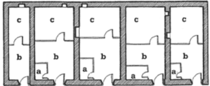
Conxunto de cinco sequeiros acaroados en As Carballeiras, Tronceda (Castro Caldelas): a. Cortello b. Cuarto e almacén de leña c. Caniceira
