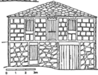
Alzado frontal
