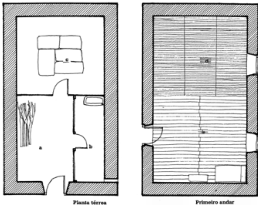
Sequeiro de dous andares con cortello e cuarto en Entrambasaugas (Castro Caldelas)
