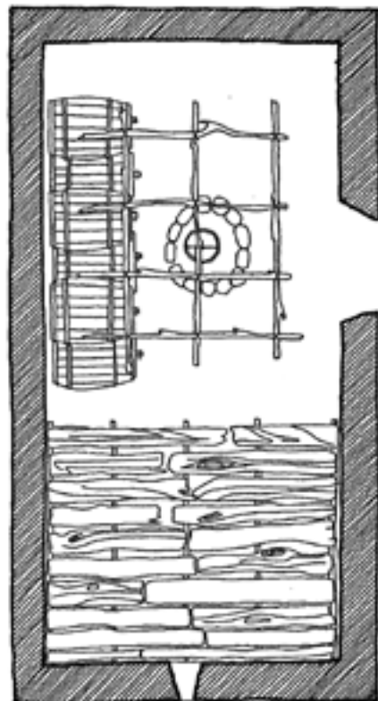
Planta
