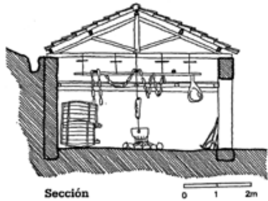
Adegavivenda con canizo en Viana do Bolo
