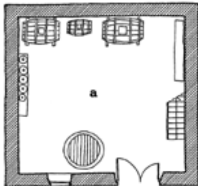
Planta térrea
