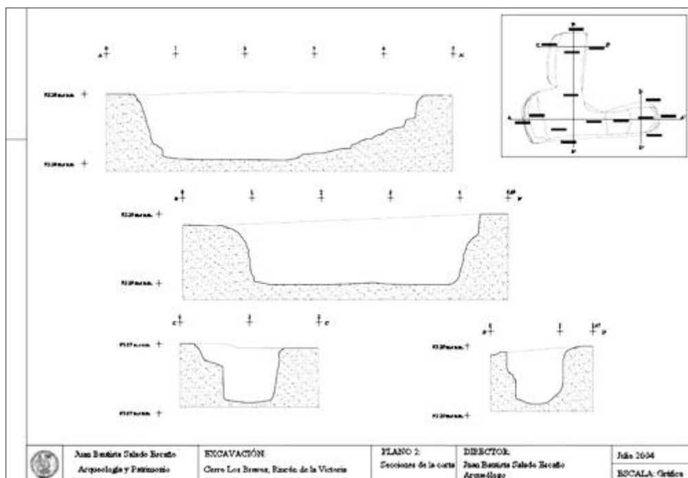
Figura 9. Plano de planta y secciones de la corta minera de cobre asociada a Bezmiliana
