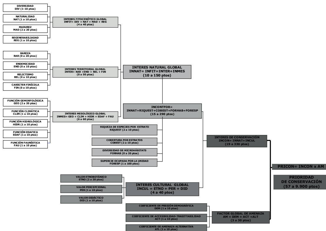
Grafico 2. Esquema del método de valoración biogeográfica LANBIOEVA
