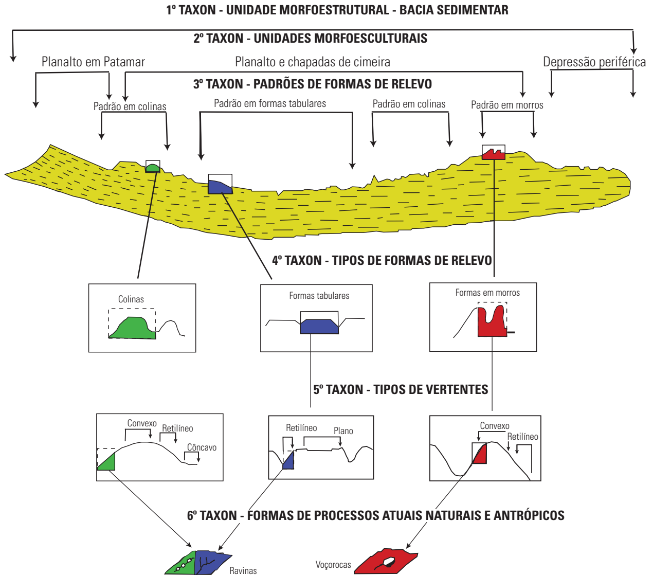
Figura 4. Unidades taxonômicas de classificação do relevo. Fonte: adaptado de Ross 1992, 22.
