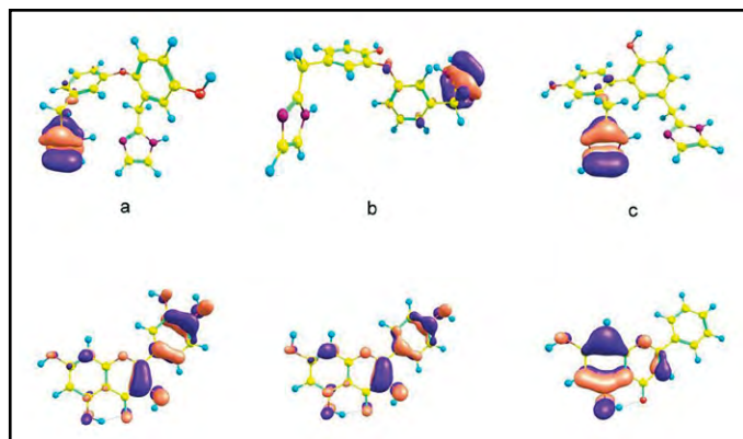
Figura 3. Orbital HOMO obtenido con B3LYP/6-31+G(d) para: a) Lepidina D, b) Lepidina E, c) Lepidina F, d) quercetina, e) camferol y f) crisina. Valores de la isosuperficie de 0.05. Elaboración propia.
