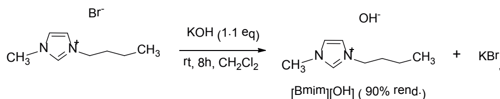
Figura 2. Síntesis del [Bmim][OH], mediante reacción de intercambio aniónico
