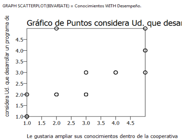
Figura. 1. Regresion lineal
