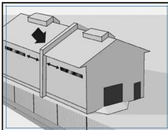
Figura 12.- Muro rompe fuegos con 15 cm de espesor tanto en las paredes como en el techo y debe sobresalir hasta una altura de 1 metro.
