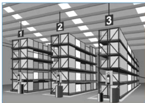
Figura 15.- Los pasillos deben ser suficientemente amplios para el tráfico peatonal y vehicular Fuente: Guías ambientales de almacenamiento y transporte
