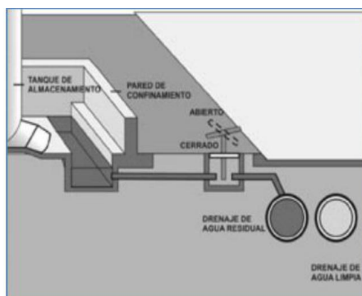
Figura 10.- Canal periférico de recolección construido de hormigón el cual se conectará con un almacenamiento y sumidero externo
