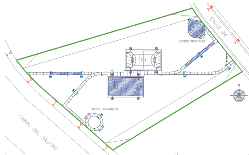
Figura 1. Plano esquemático del parque seleccionado como caso de estudio, en donde se localizan los puntos de luz existentes.
