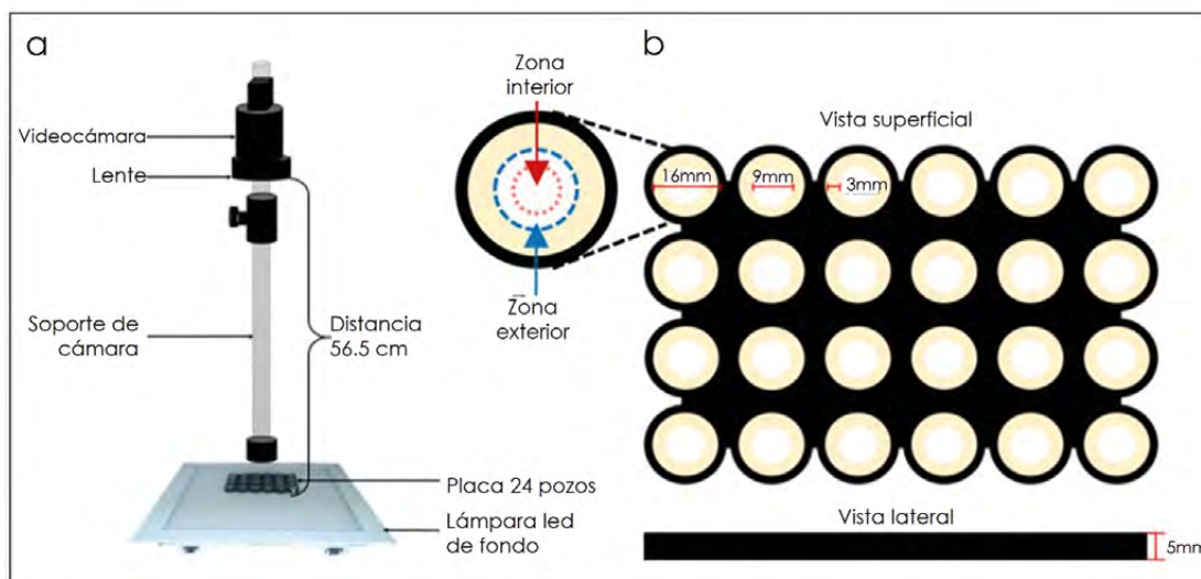
Figura 2. Diseño de equipo y material para el análisis locomotor en larvas de pez cebra. (a) Montaje para videograbación de placas, (b) placas de 24 pocillos con delimitación de agar en la periferia de los pocillos. Elaboración propia.
