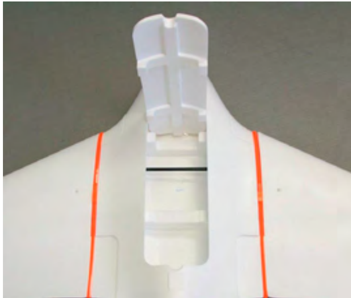
Figura 7: Detalle bahía interna del Skywalker X8 donde pueden alojarse dispositivos improvisados (IED) Fuente: Onedrone.com
