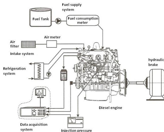
Figura. 1. Configuración experimental. Fuente. Referencia [34].
