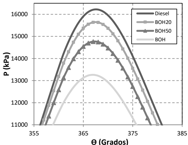
Figura 4. Presión versus ángulo de giro del cigüeñal para mezclas diesel/bio-oil hidrotratado con el motor operando a alta carga y 2000 rpm. Fuente. Autores.
