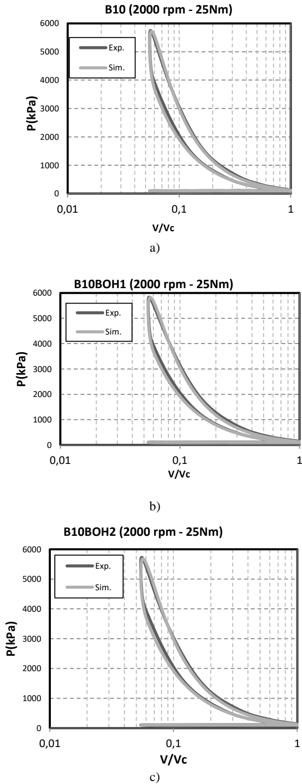
Figura 3. Comparación entre las curvas experimentales y simuladas del motor Isuzu a 2000 rpm y 25 N.m. a) Motor alimentado con combustible B10, b) Motor alimentado 99% de combustible B10 y 1% de bio-oil hidrotratado, c) Motor alimentado 98% de combustible B10 y 2% de bio-oil hidrotratado. Fuente. Autores.
