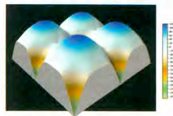
Figura 6. Variación de la constante de acoplamiento J(^{19}\text{F}-^{19}\text{F}) del dímero del fluoruro de hidrógeno con la geometría
