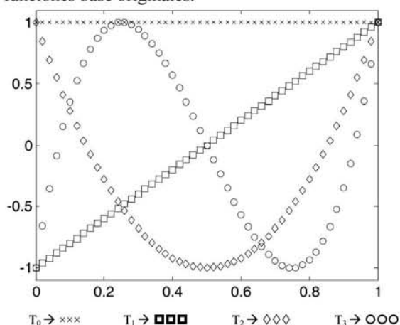
Figura 1. Polinomios de Chebyshev
