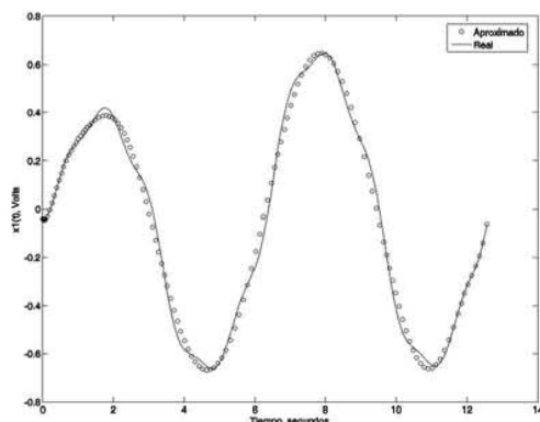
Figura 3. Solución de x_1 simulada con 16 polinomios
