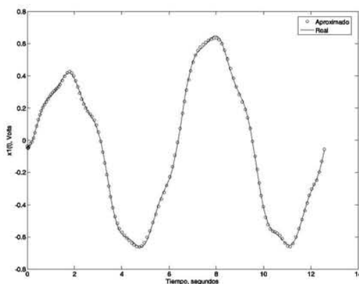
Figura 4. Solución de x_1 simulada con 32 polinomios
