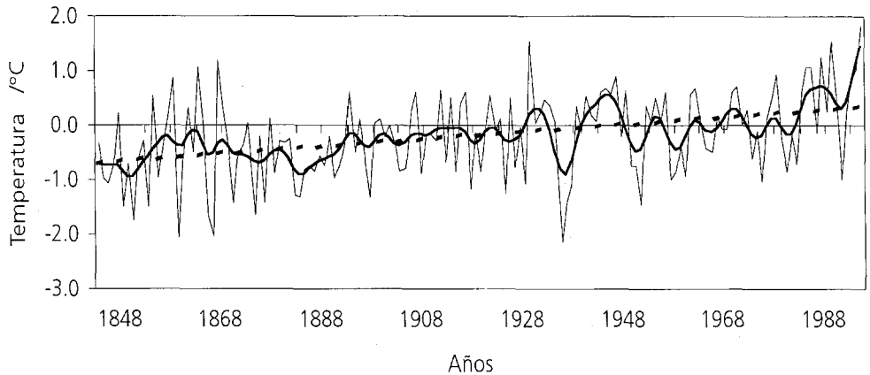
Figura 10. Temperaturas medias anuales de la República Checa 1848-2000, expresadas como anomalías sobre el período de referencia 1961-1990. Serie Nacional. Suavizado de 10 años con filtro de paso bajo de Gauss. La línea quebrada indica la tendencia lineal 1848-2000.
