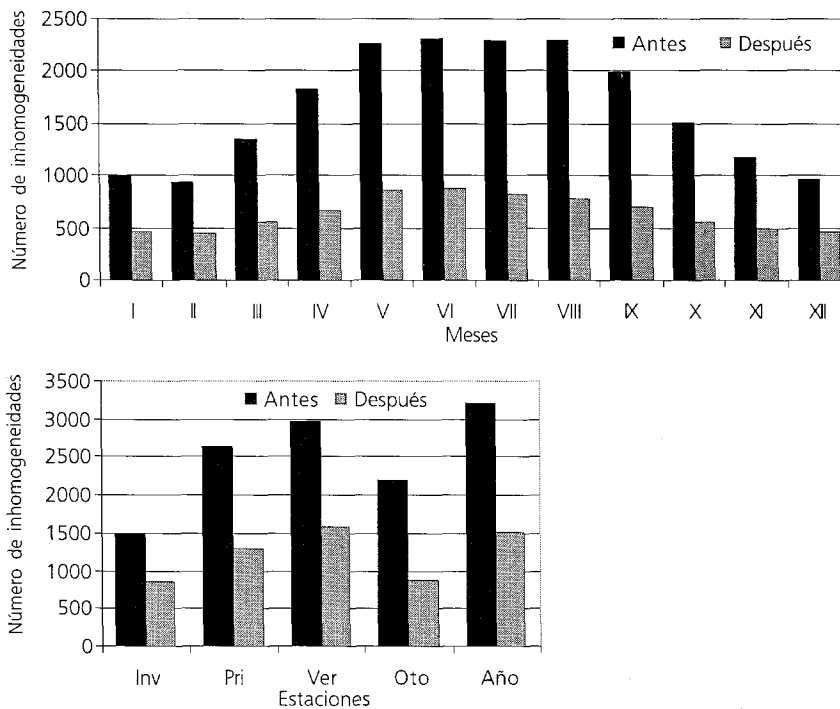
Figura 5. Número de inhomogeneidades significativas (mensuales, estacionales y anuales) detectadas antes y después del proceso de homogeneización. Número total de series comprobadas: antes de la corrección, en torno a 41.000, después de la corrección, en torno a 36.000 series ( \alpha=0.05 ).
