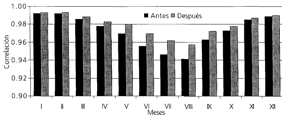
Figura 7. Mediana del coeficiente de correlación previo y posterior al homogeneizado entre las estaciones candidatas y de referencia (231 series ajustadas).
