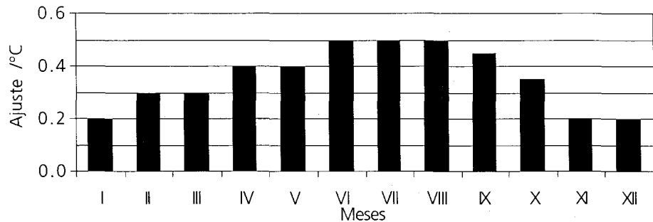
Figura 6. Valor de la mediana de las cantidades ajustadas en las series. Valores absolutos (°C). Series ajustadas 231.
