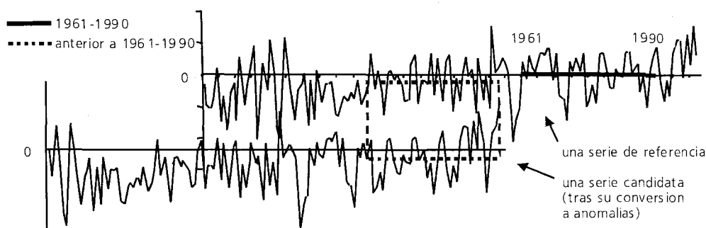
Figura 4. Ejemplo de conversión de una serie anterior a 1961-1990 en anomalías sobre el período citado. La serie de referencia (superior en la figura) y la serie candidata (inferior) al convertirse en anomalías sobre 1961-1990 pueden ser comparadas por tener el mismo promedio en algún periodo consecutivo de 30 años.
