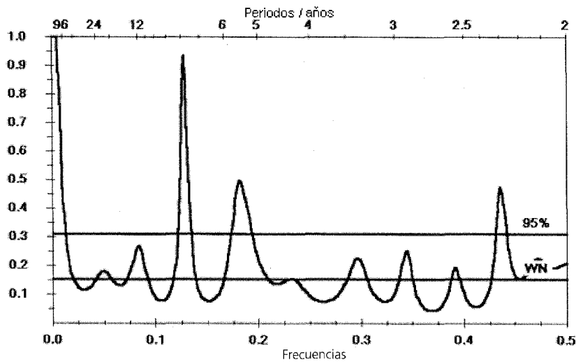
Figura 11. Análisis espectral (MESA) de los valores de temperatura media anual de la República Checa, 1848-2000, m=30 .
