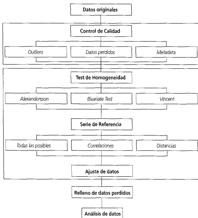
Figura 3. Esquema general del método de procesado de datos climáticos empleado en el presente estudio.
