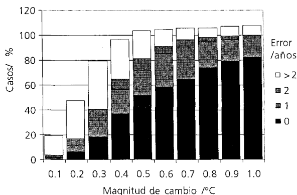
Figura 2. Porcentaje de casos detectados según distintas magnitudes de cambio introducidas artificialmente y error de la detección del año correcto. Extractado a partir de información obtenida de 950 series y SNHT, con \alpha=0.05 .
