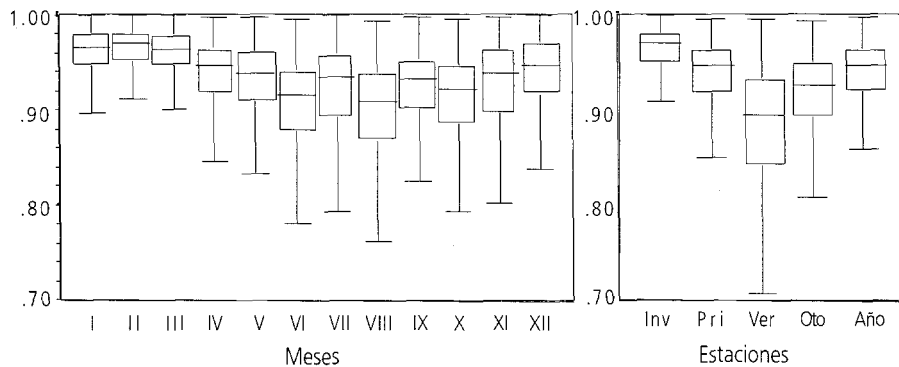
Figura 9. Coeficientes de correlación (box plot) mensual, estacional y anual entre todas las series. Cada caso representa 9187 valores.
