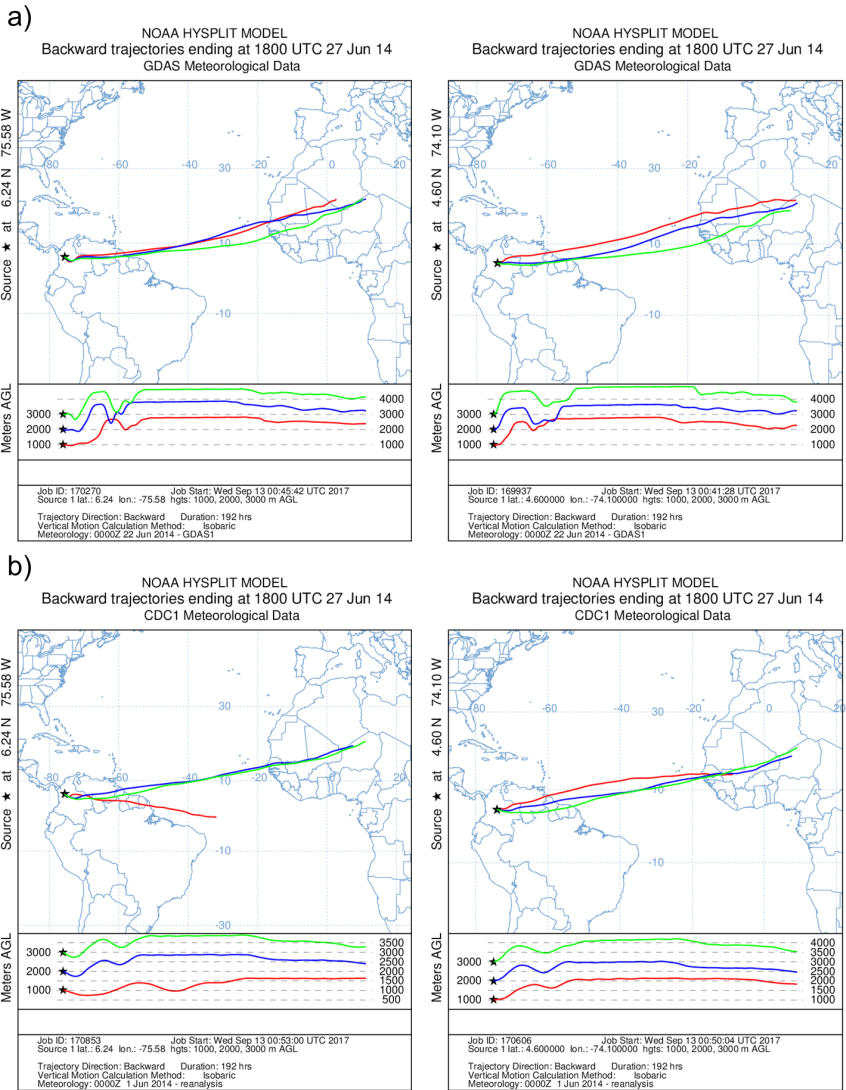
Figura 7. Origen de trayectorias de masas de aire con Hysplit para el 27 de junio de 2014 a) base meteorológica GDAS 1 , b) base meteorológica Reanalysis. Los receptores son Medellín (columna izquierda) y Bogotá (columna derecha) a las 18 UTC a 1000, 2000 y 3000 metros sobre el nivel del suelo.
