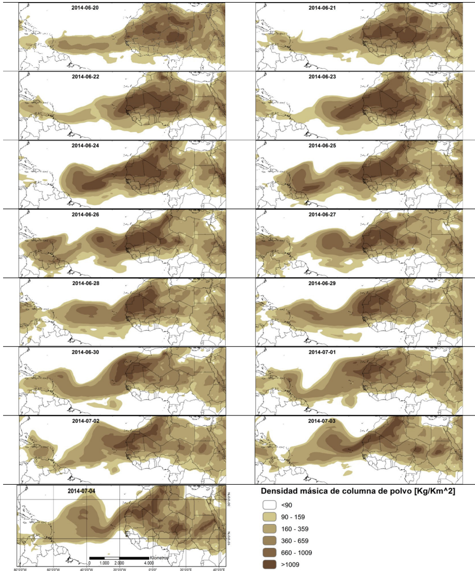
Figura 5. Transporte transatlántico de polvo africano desde el 20 de junio al 4 de julio de 2014.
