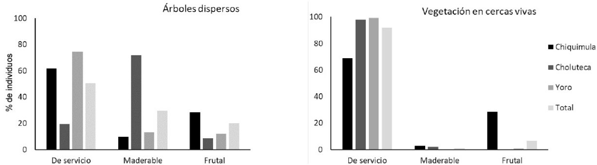
Figura 3. Uso de árboles dispersos registrados en las parcelas de granos básicos (n=1686) y las cercas vivas (n=3143) en fincas de pequeños agricultores de granos básicos en tres paisajes centroamericanos, uno en Guatemala (Chiquimula) y dos en Honduras (Choluteca y Yoro). Julio 2014 - junio 2015.
