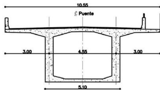
Figura 2. Sección transversal de la viga cajón del puente Gómez Ortiz. Fuente: [2].
