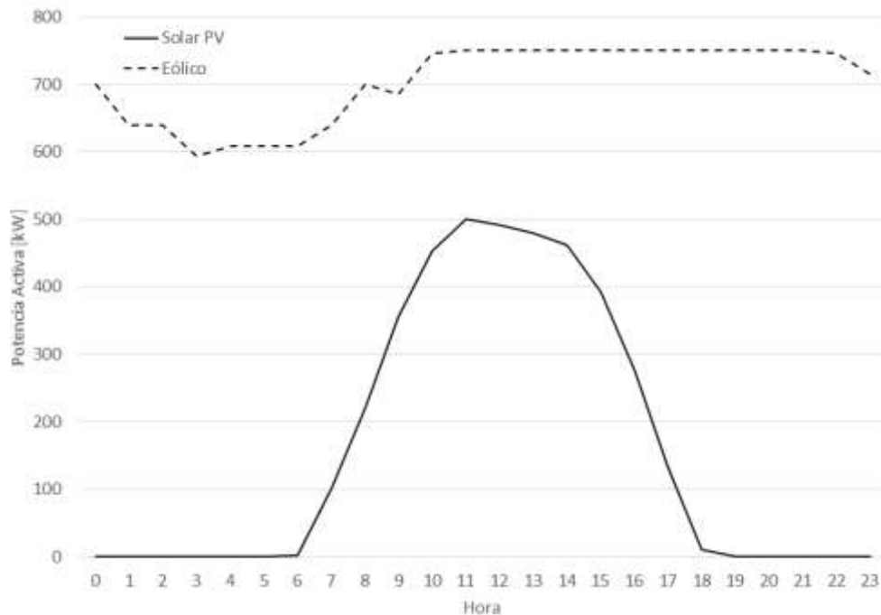
Figura 16. Comportamiento de la generación eólica y fotovoltaica Fuente: elaboración propia.
