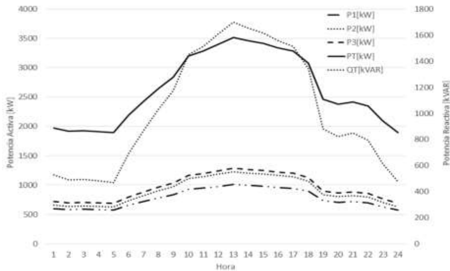
Figura 13. Comportamiento de la potencia activa y reactiva del sistema IEEE original Fuente: elaboración propia.
