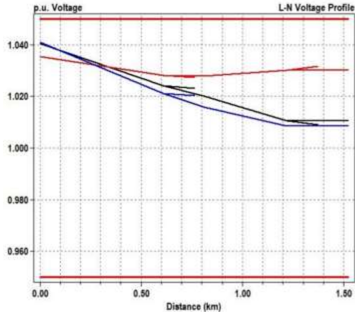
Figura 14. Perfil de tensiones para el sistema IEEE original
