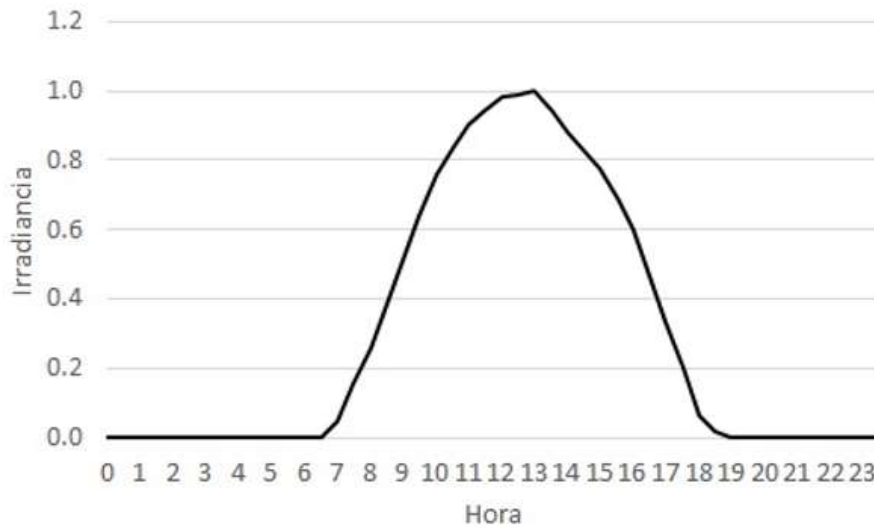
Figura 10. Curvas de irradiancia usada para modelar la generación fotovoltaica Fuente: Elaboración propia.
