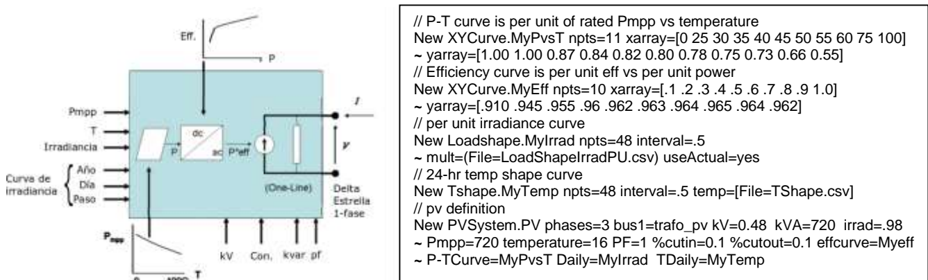
Figura 9. Diagrama de bloques y declaración del sistema de generación solar [14].
