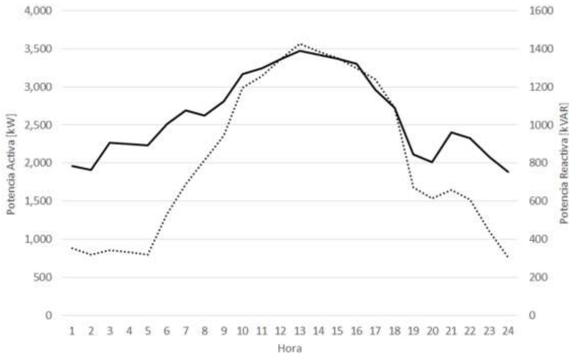
Figura 18. Suministro de energía activa y reactiva de la red IEEE modificada Fuente: elaboración propia.
