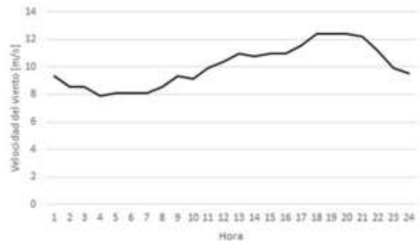
Figura 12. Curva de velocidad del viento y código de programación del generador eólico.
