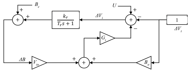
Figura 2. Modelo del SVC planteado
