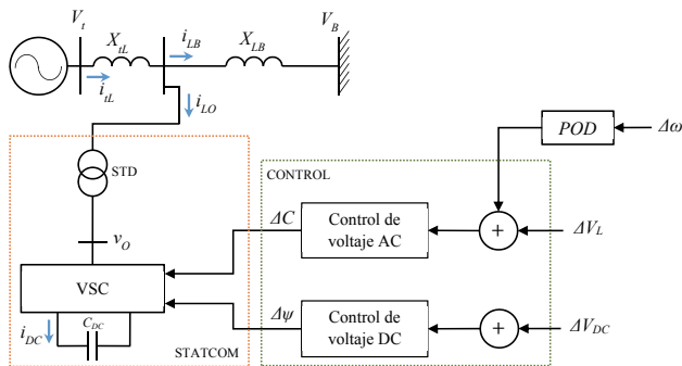
Figura 4. STATCOM instalado en el sistema SMIB
