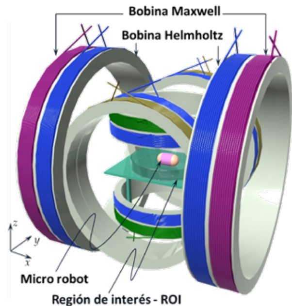
Figura 3. Diagrama sistema actuador electromagnético para micro-robots
