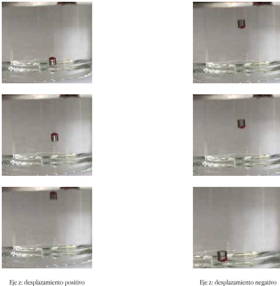
Figura 8. Desplazamiento del micro-robot bobinas Helmholtz y Maxwell, Eje: z, 90o.
