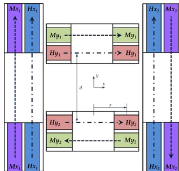
Figura 5. Diagrama esquemático del sistema actuador electromagnético (EMA) plano x-y .
