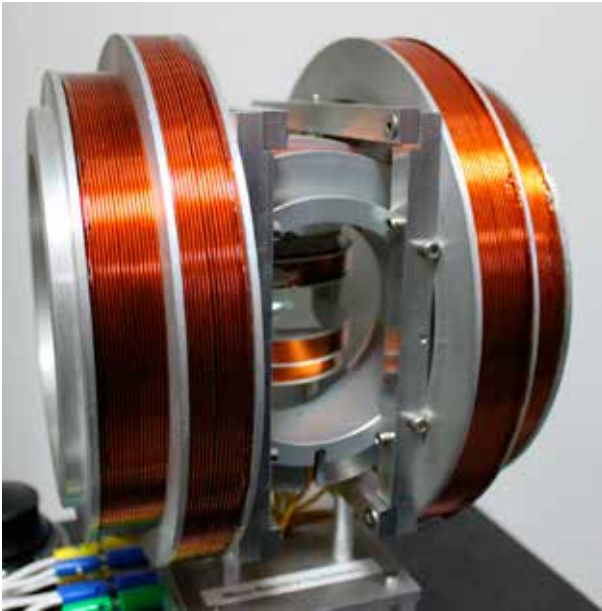
Figura 6. Actuador Electromagnético para micro-robots
