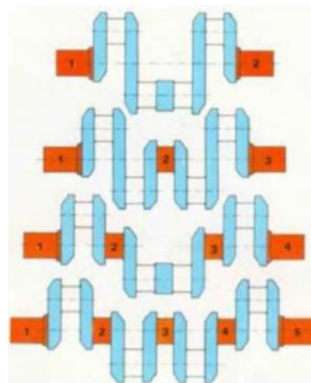
Figura 1. Cigüeñal equilibrado estáticamente (Sánchez, 2016)
