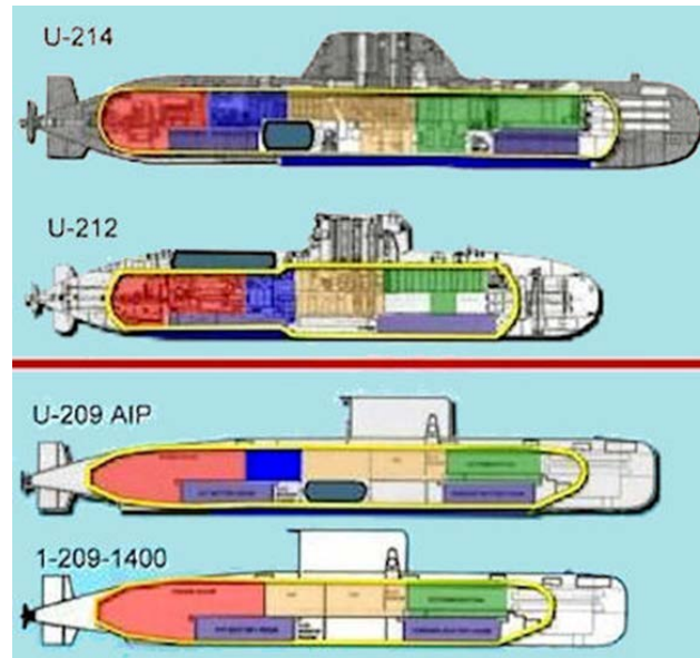
Figura 11. Variantes de submarinos de ThyssenKrupp Marine Systems (Internet)
