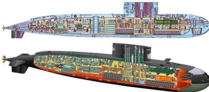
Figura 5. Submarino clase Kilo 636M (Rubin Central Design Bureau)
